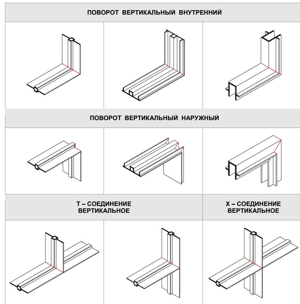
Возможные виды фасонных элементов
