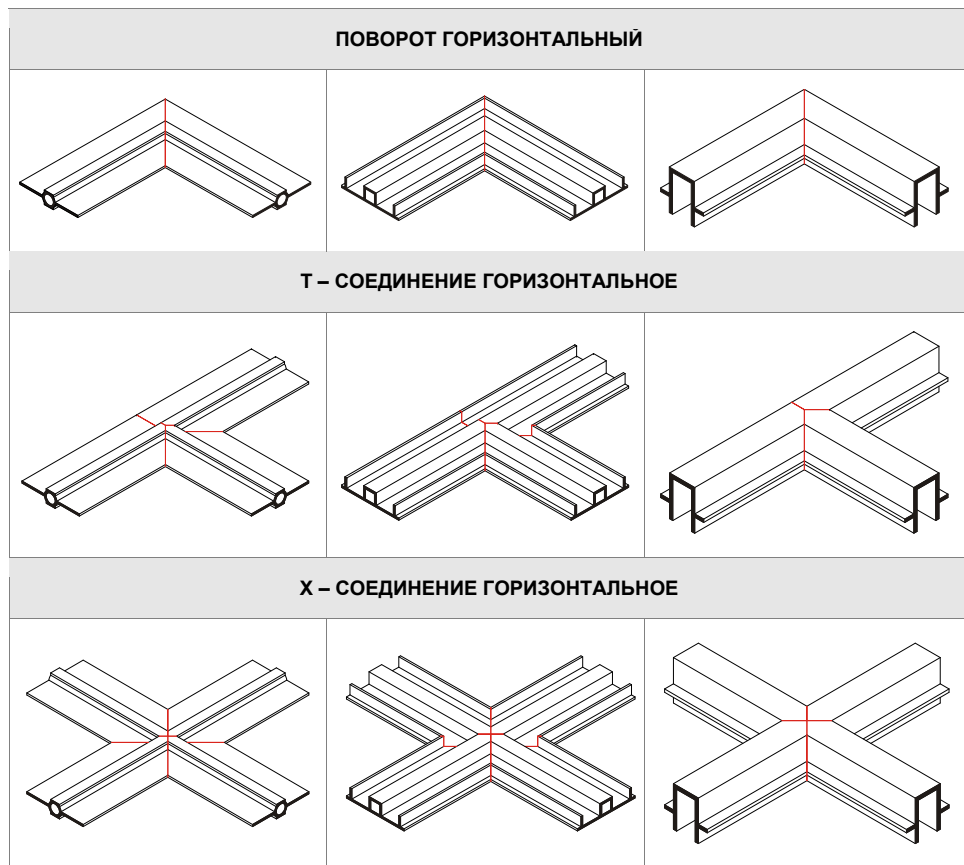
Возможные виды фасонных элементов
